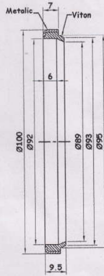
ITEM - 2 WIPER SEAL Qty Reqd : 1 No.
