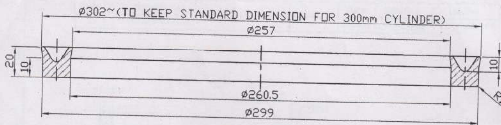
ITEM 1 PISTON SEAL Qty. Reqd : 2Nos.
